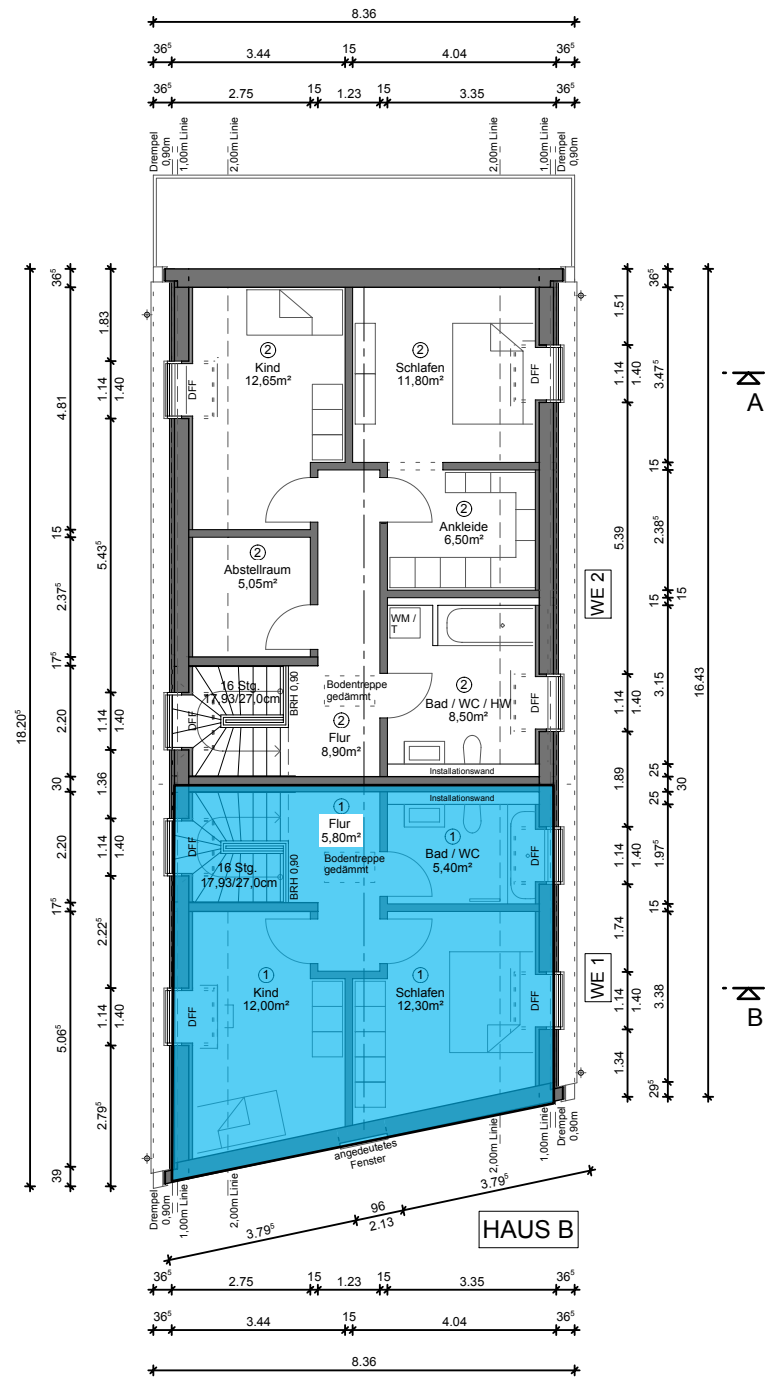
GRUNDRISS DACHGESCHOSS
